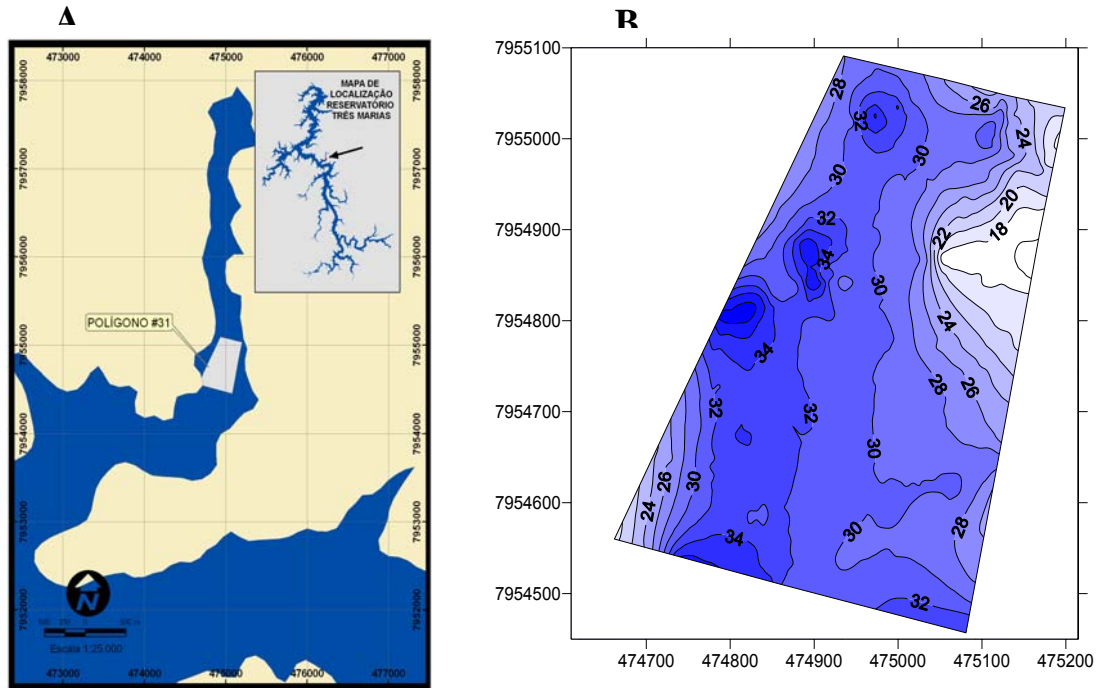
Figura 3 – Mapa de localização (A) e mapa batimétrico (metros) (B) da Área Aqüícola 31 no Parque Aqüícola Indaiá 1, reservatório de Três Marias (MG).
