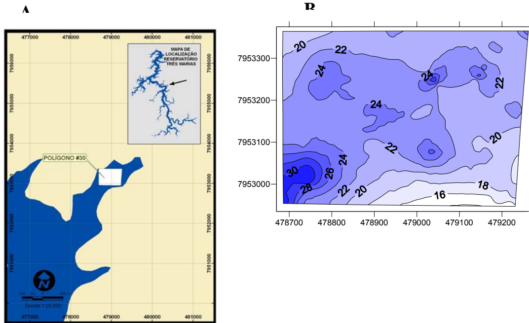
Figura 2 – Mapa de localização (A) e mapa batimétrico (metros) (B) da Área Aqüícola 30, no Parque Aqüícola Indaiá 1, reservatório de Três Marias (MG).
