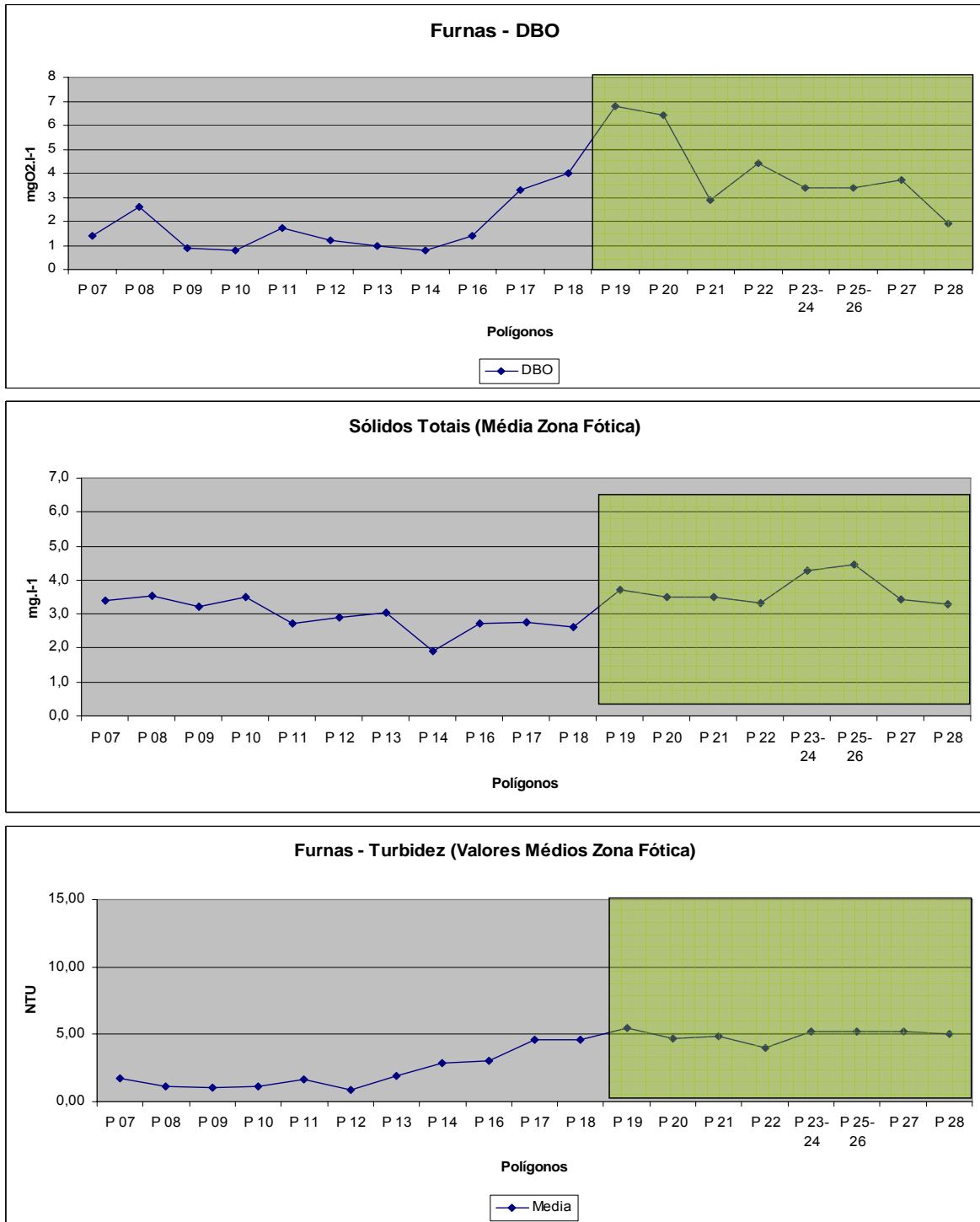
Figura 88 – Turbidez, sólidos e DBO em diferentes áreas aquícolas demarcadas no reservatório de Furnas. Coletas: fevereiro de 2007.
