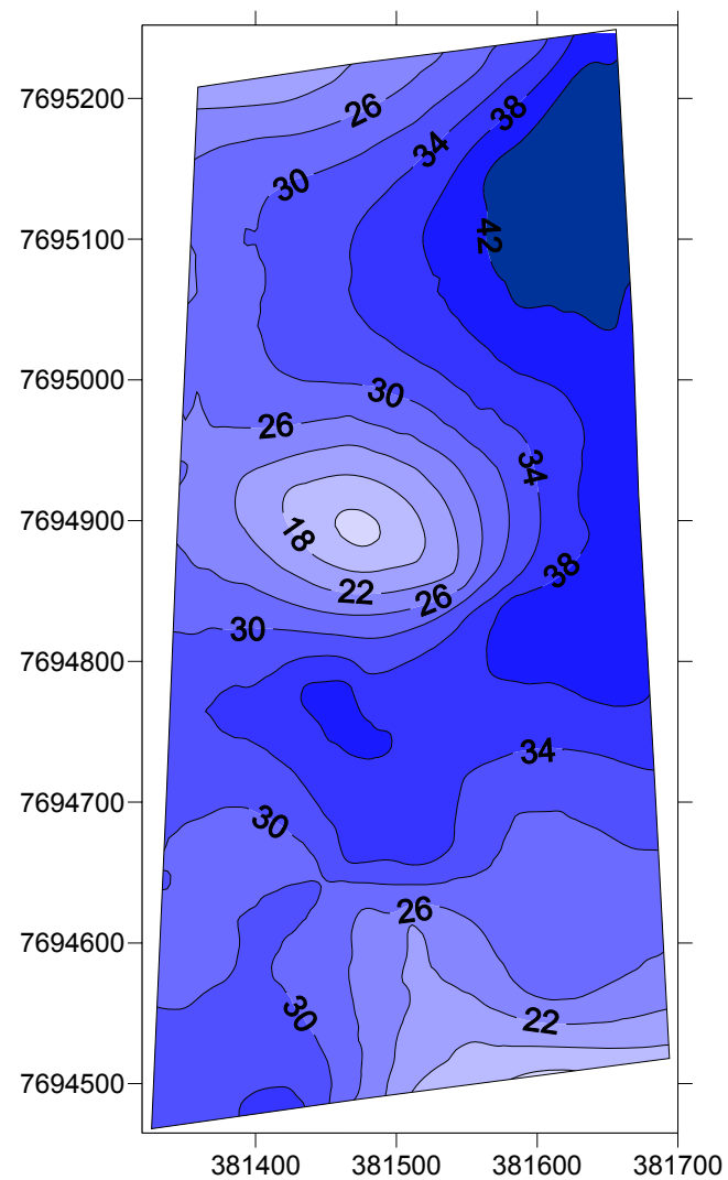
Figura 4 – Mapa de localização (A) e mapa batimétrico (metros) (B) do polígono 16 no reservatório de Furnas (MG).
