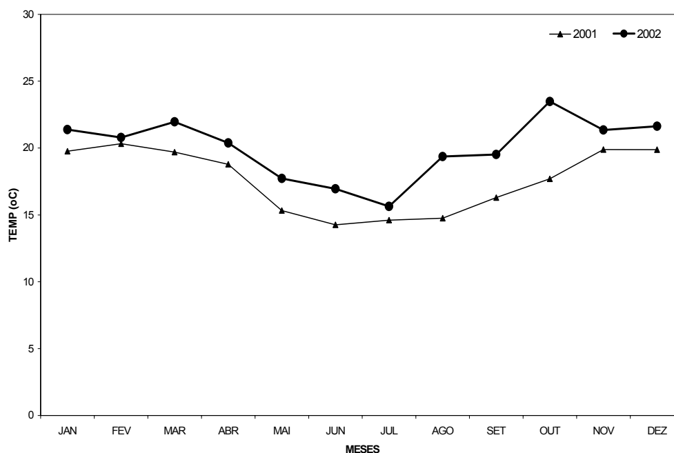
Figura 14 – Distribuição anual de temperatura média do ar, na estação MTLC1, para os anos de 2001 e 2002.
