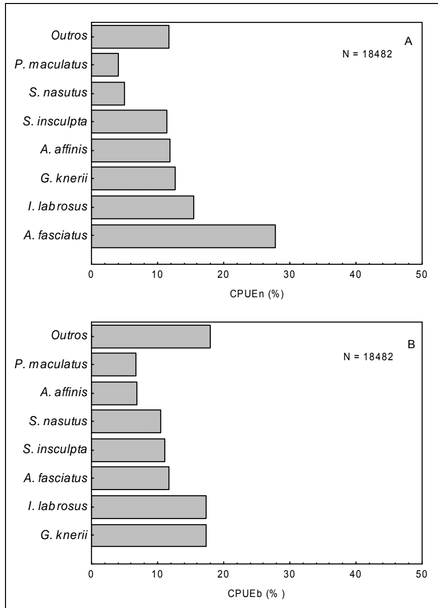
Figura 28 – Percentual de capturas em número (A) e biomassa (B) para as espécies mais capturadas no reservatório de Furnas, levando-se em conta coletas bimestrais entre agosto/92 e junho/94. CPUE = Capturas por unidade de esforço em número (n) e biomassa (b); N = número de exemplares utilizados (Fonte: Santos, 1999).
