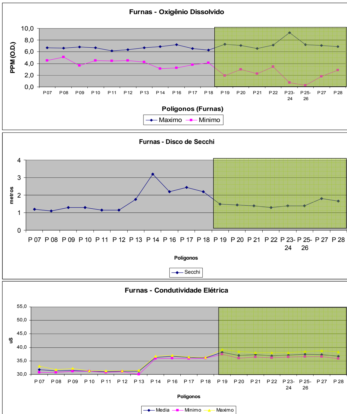
Figura 87 – Oxigênio dissolvido (superfície e fundo), transparência da água e condutividade elétrica (superfície e fundo) nas áreas aquícolas demarcadas no reservatório de Furnas, MG.
