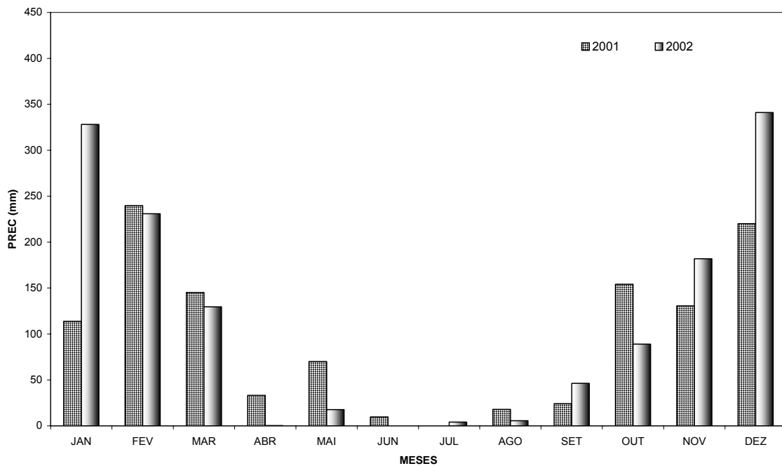
Figura 18 – Distribuição mensal de precipitação na estação MTCL, para os anos de 2001 e 2002.
