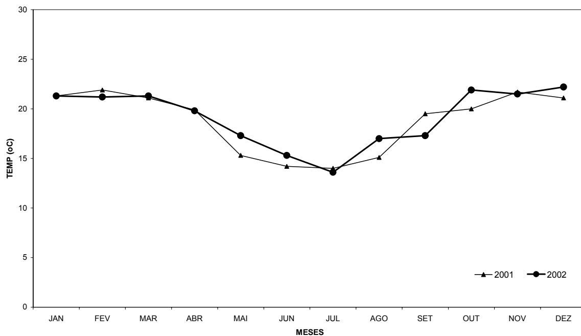
Figura 19 – Distribuição anual de temperatura média do ar, na estação MTCL, para os anos de 2001 e 2002.
