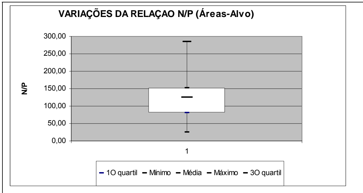
Figura 7 – Variação dos valores da Relação N:P (Nitrogênio Total e Fósforo Total, by weight) para os dados limnológicos do levantamento das Áreas Alvo do Reservatório de Furnas, realizado em 2006. (N=40).
