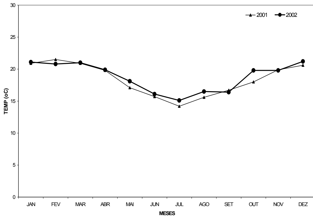
Figura 25 – Distribuição anual de temperatura média do ar, na estação MTIT, para os anos de 2001 e 2002.
