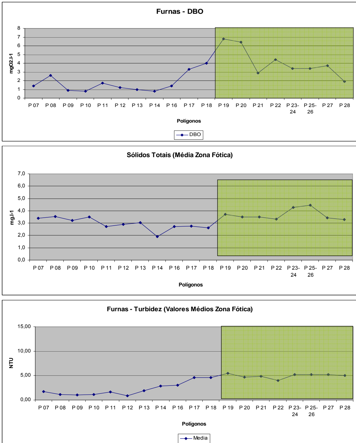
Figura 91 – Turbidez, sólidos e DBO em diferentes áreas aquícolas demarcadas no reservatório de Furnas. Coletas: fevereiro de 2007.
