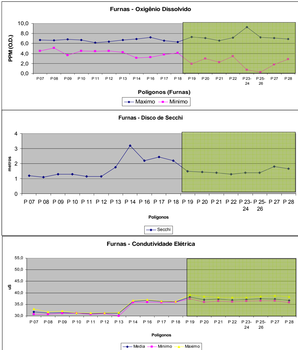
Figura 90 – Oxigênio dissolvido (superfície e fundo), transparência da água e condutividade elétrica (superfície e fundo) nas áreas aquícolas demarcadas no reservatório de Furnas, MG.
