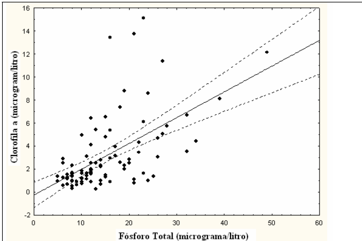
Figura 8 – Regressão linear (clorofila X fósforo): \text{clorofila} = -0,243 + 0,224 * \text{Fósforo} ; N = 94 ; R^2 = 0,33 r = 0,58 .
