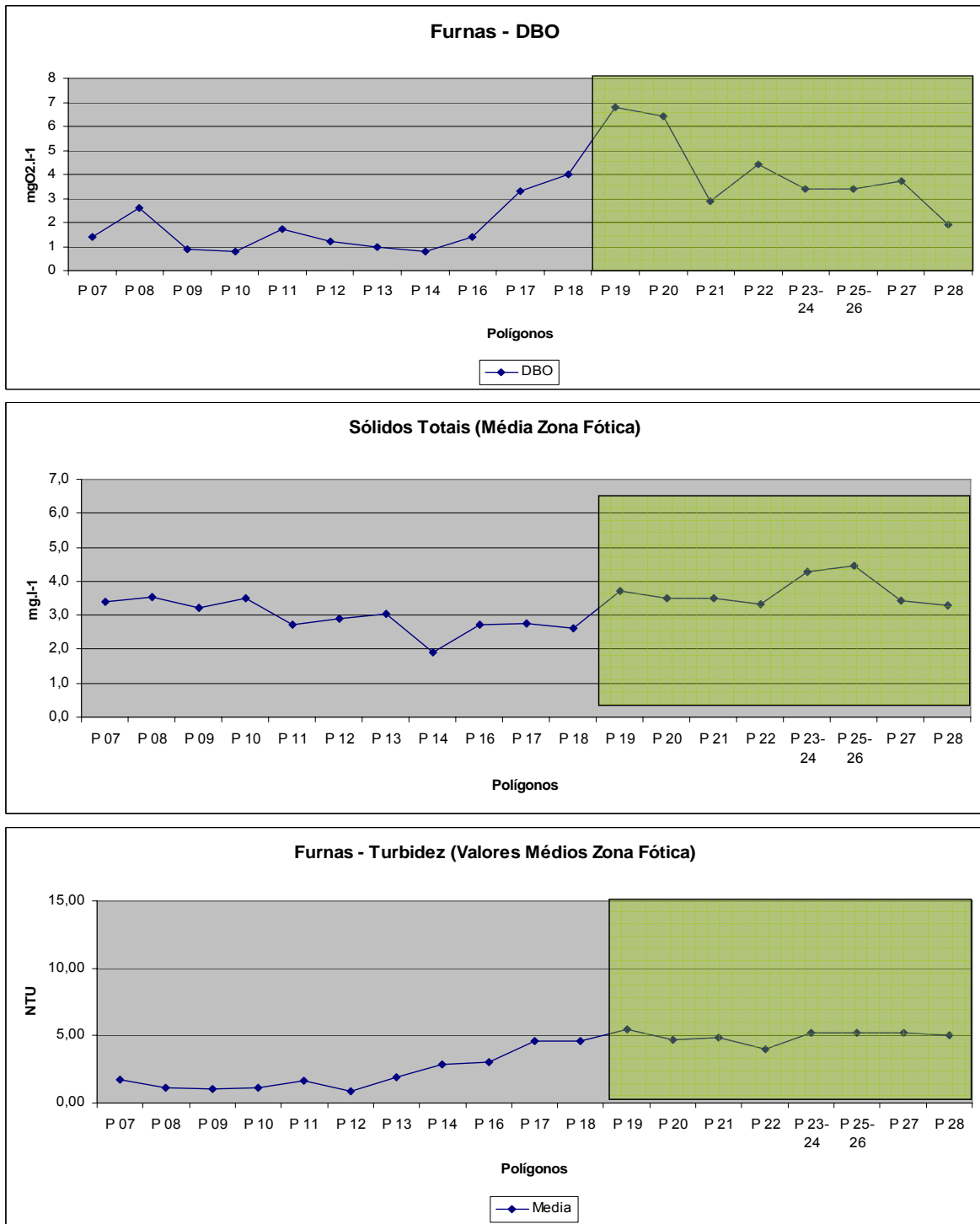
Figura 94 – Turbidez, sólidos e DBO em diferentes áreas aquícolas demarcadas no reservatório de Furnas. Coletas: fevereiro de 2007.
