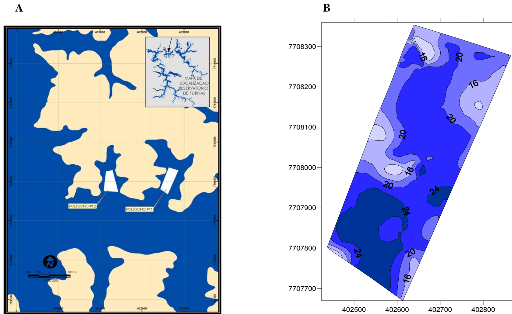
Figura 3 – Mapa de localização (A) e mapa batimétrico (metros) (B) do polígono 11 no reservatório de Furnas (MG).
