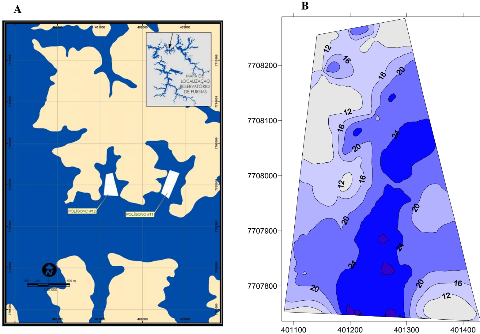
Figura 5 – Mapa de localização (A) e mapa batimétrico (metros) (B) do polígono 12 no reservatório de Furnas (MG).
