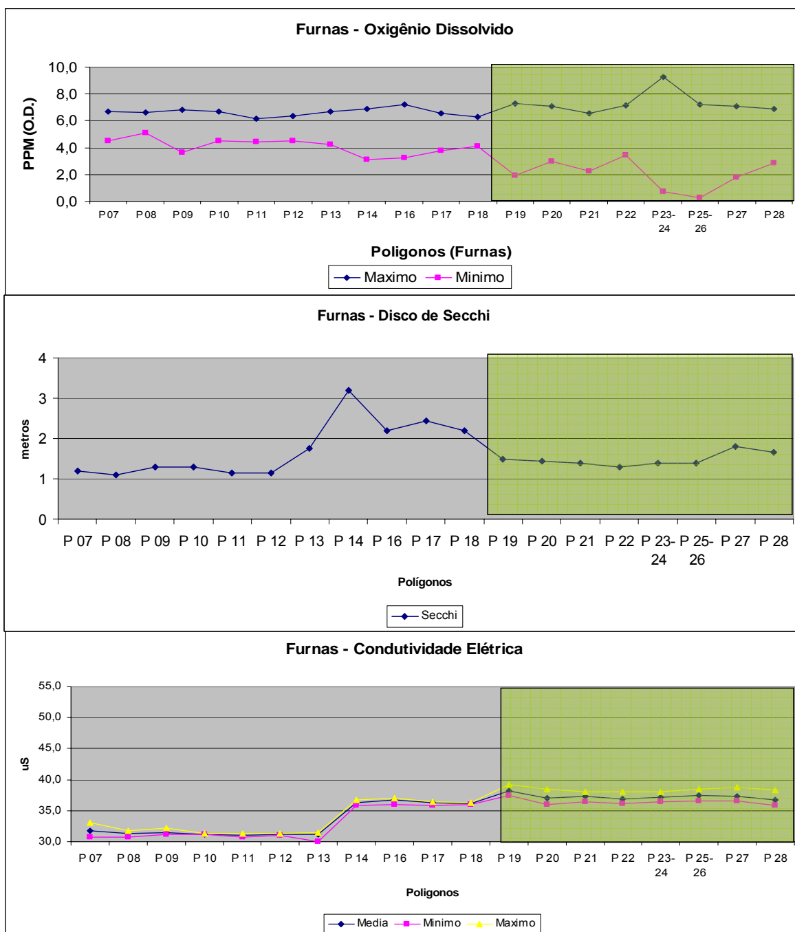
Figura 93 – Oxigênio dissolvido (superfície e fundo), transparência da água e condutividade elétrica (superfície e fundo) nas áreas aquícolas demarcadas no reservatório de Furnas, MG.
