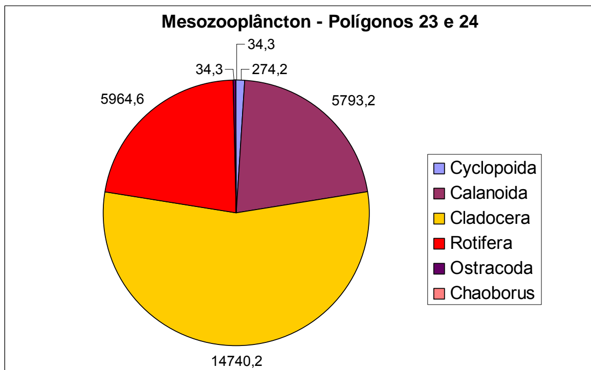
Figura 27 – Composição e densidades (ind/m 3 ) dos principais grupos de organismos zooplanctônicos no polígono 23 e 24, parque aqüícola do Barranco Alto-2, reservatório de Furnas, MG.
