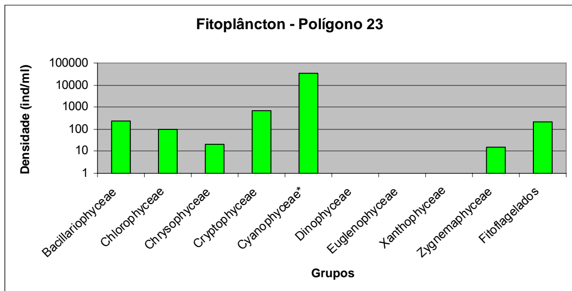
Figura 26 – Densidades dos principais grupos de organismos fitoplanctônicos no polígono 23, Parque Aquícola do Barranco Alto-2, reservatório de Furnas.
