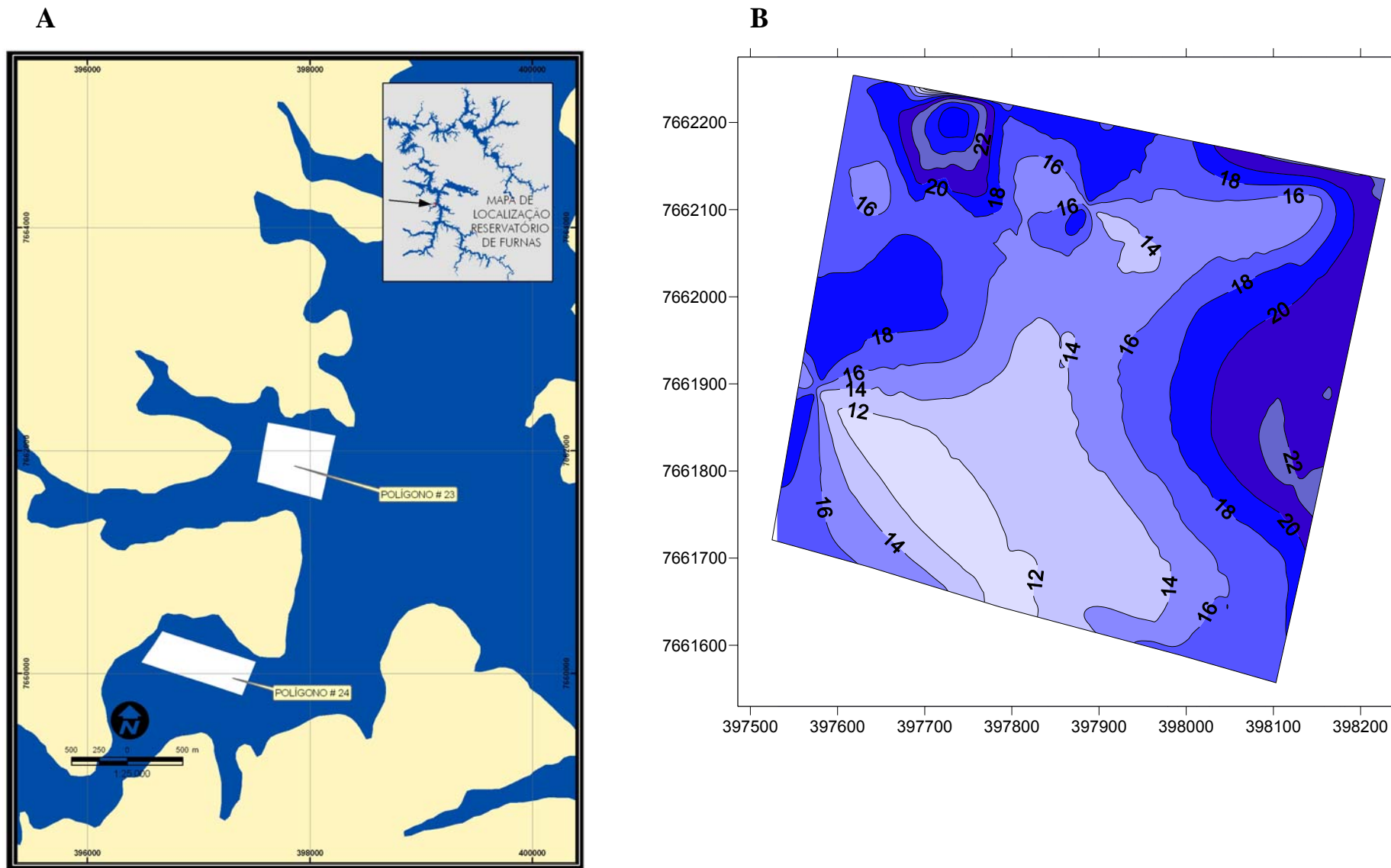
Figura 3 – Mapa de localização (A) e mapa batimétrico (metros) (B) do polígono 23 no reservatório de Furnas (MG).
