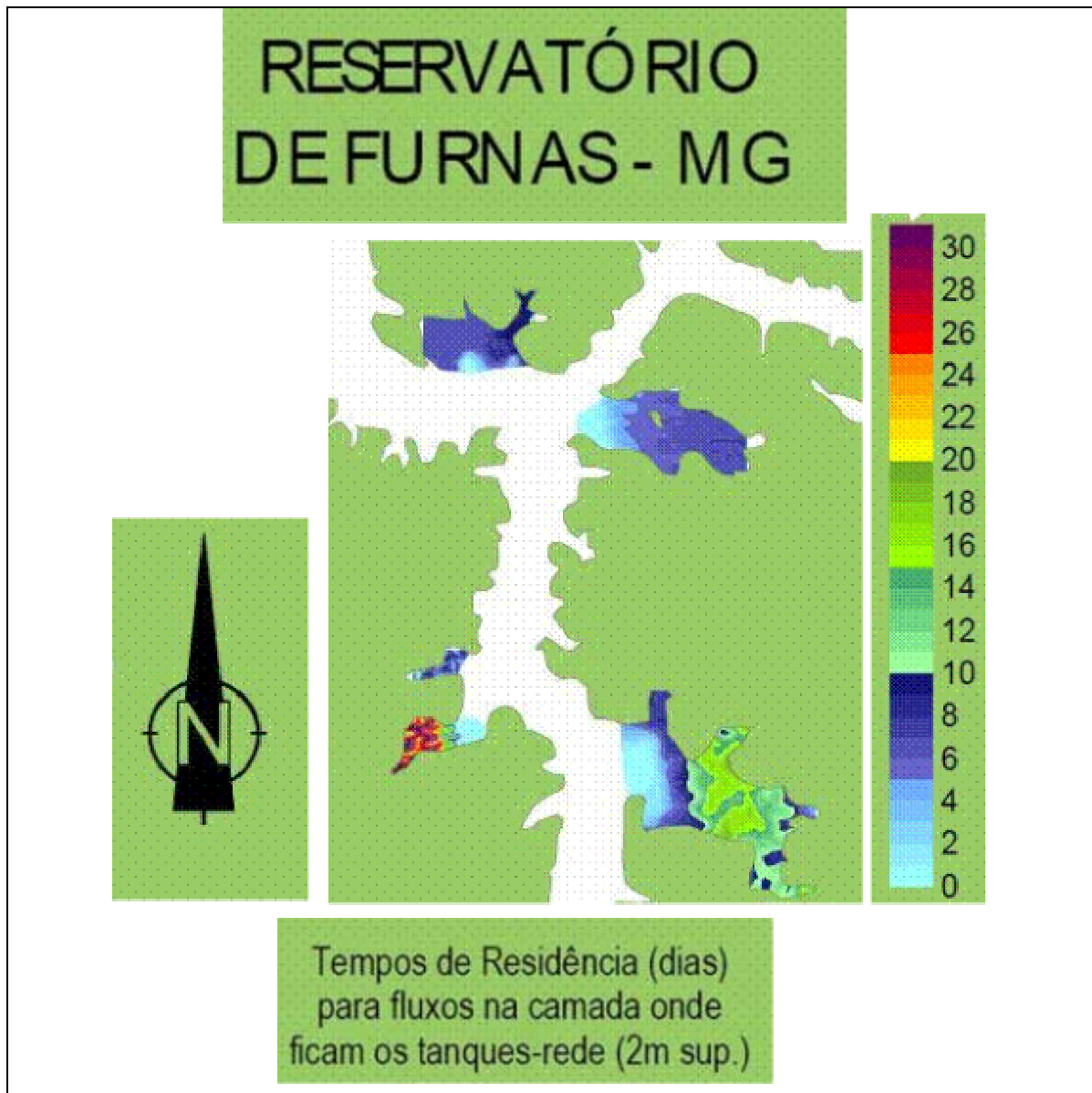
Figura 9 – Tempos de residência na camada superficial da água das áreas aquícolas 23, 24, 25 e 26 pertencentes aos parques aquícolas do Barranco Alto-1 e 2, reservatório de Furnas. Simulações feitas pelo sistema SISBAHIA, COPPETEC/UFRJ.
