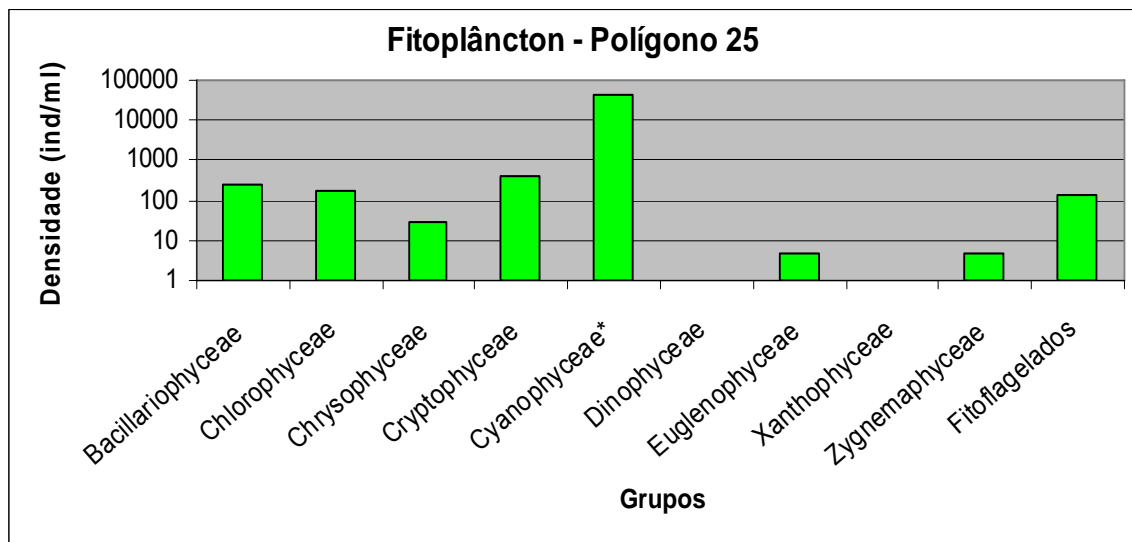
Figura 26 – Densidades dos principais grupos de organismos fitoplanctônicos no polígono 25, Parque Aquícola do Barranco Alto-1, reservatório de Furnas.
