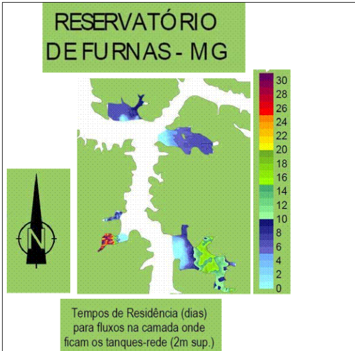
Figura 9 – Tempos de residência da camada superficial da água nos parques aquícolas do Campo do Meio, Barranco Alto 1 e 2, reservatório de Furnas, MG. Simulações feitas pelo sistema SISBAHIA, COPETTEC/UFRJ.
