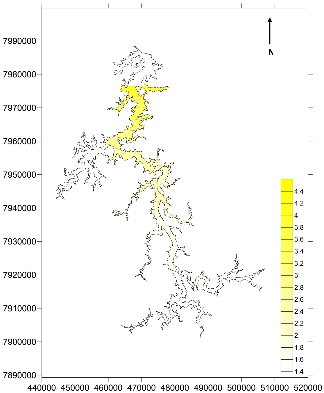
Figura 16 – Mapa temático de profundidade do Secchi (m) - Reservatório de Três Marias.
