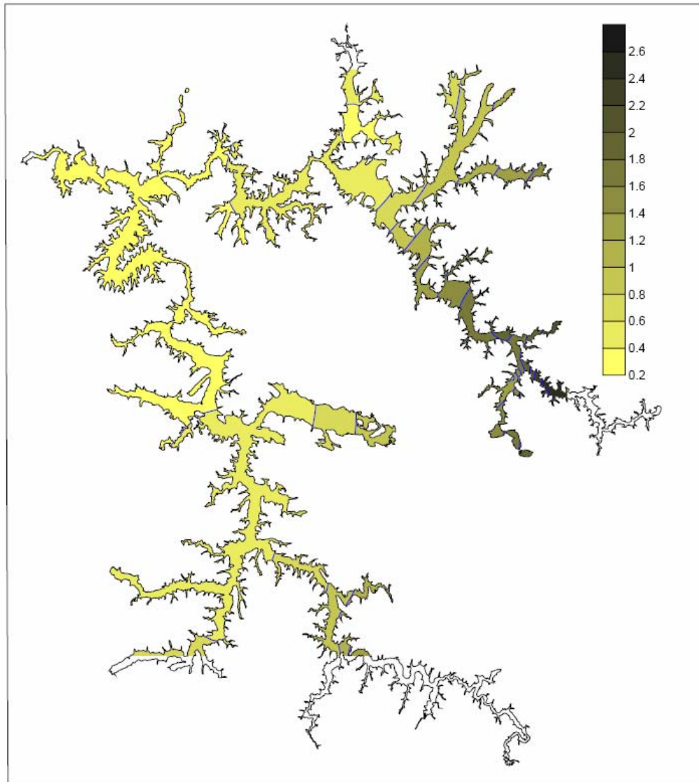
Figura 19 B - Padrões espaciais (interpolação obtida com o programa Sufer 8.0) mostrando um aumento dos coeficientes de extinção da radiação fotossinteticamente ativa (PAR, 430-700 nm) em direção às estações de montante, nos dois sub-eixos do Reservatório de Furnas (Sapucai e Grande), entre fevereiro e março de 2006.
