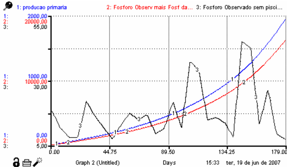
Figura 6.7 - Variação da “Produção Primária”, do “Fósforo observado + Fósforo proveniente da ração” e do “Fósforo na água”, simulada SEM DILUIÇÃO pelo modelo CRITITA para Três Marias.
