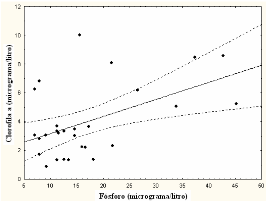
Figura 3 – Regressão linear clorofila x fósforo para o reservatório de Três Marias (superfície). Dados coletados entre os anos de 2001-1006. N=28; r = 0,49 ; R^2 = 0,25 .
