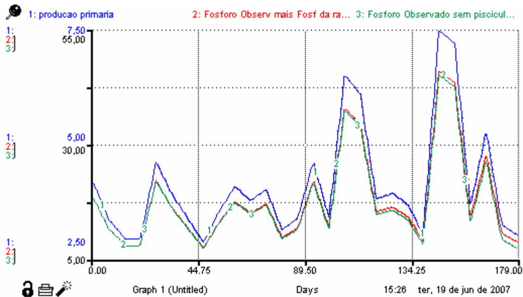
Figura 6 - Variação da “Produção Primária”, do “Fósforo observado + Fósforo proveniente da ração” e do “Fósforo na água”, simulada pelo modelo CRITITA para Três Marias. Note diferenças na escala de valores.
