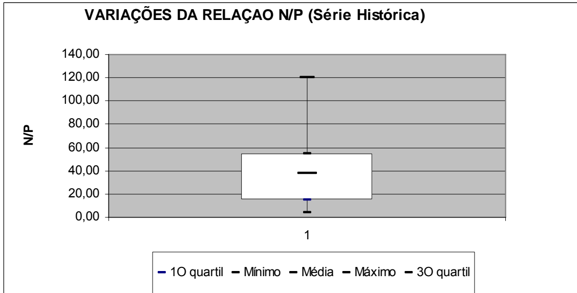
Figura 1: Variação dos valores da Relação N:P (Nitrogênio Total e Fósforo Total, by weight) para os dados limnológicos do monitoramento do Reservatório de Três Marias, para o período de 2001 a 2006, considerando simultaneamente as Estações de Amostragem M1, M3, M4, M5 e M6, monitoradas pelo Convênio CEMIG/CODEVASF(N=48).
